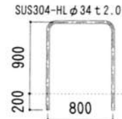
④屋外U形手摺
